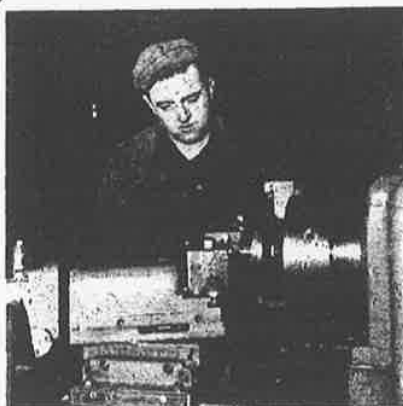
M. Blouin - 250 HN semi rompu avec appareil ad- ditionnel - Reproduction d'une roue de 76 dents.
